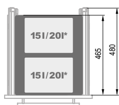
Фасад 60 NL=480
