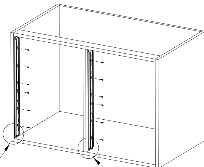
montaż listew w korpusie
